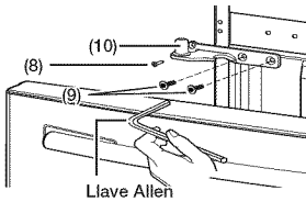
Llave Allen
